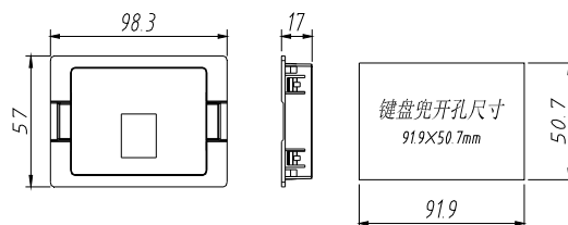
GD10 系列外引键盘外形尺寸
