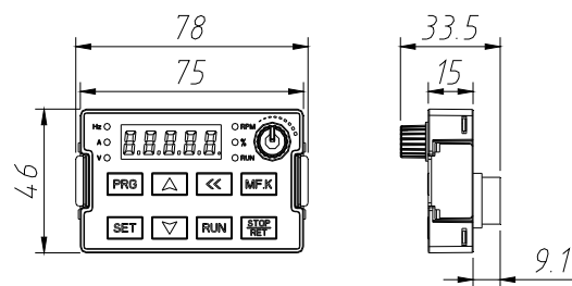
GD10 系列外引键盘外形尺寸
