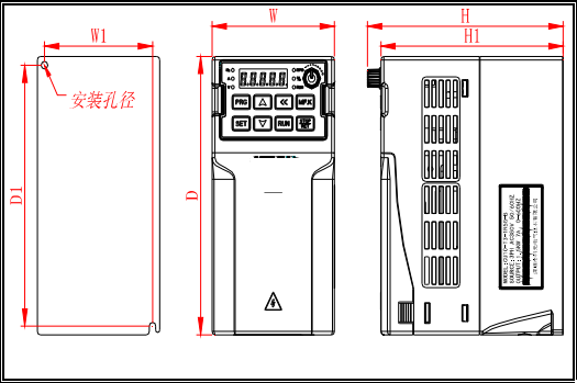
变频器及键盘的外形尺寸
