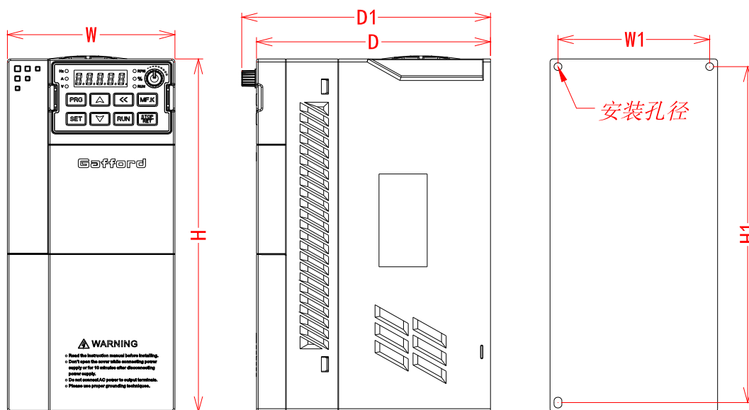
GD600 0.75G-22G 外型及安装孔位尺寸
