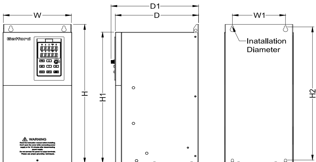
GD600 30G-400G 外型及安装孔位尺寸
